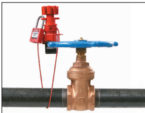
Use el accesorio de cable para bloquear válvulas de compuerta.
