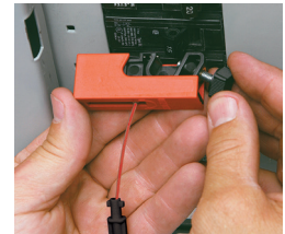
2. Coloque el dispositivo de bloqueo en el interruptor y póngalo en posición de bloqueo.
