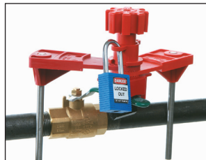
Use dos brazos de bloqueo para bloquear válvulas de 3, 4 o 5 vías, o para bloquear válvulas en la posición de encendido, apagado.
