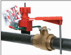
Use un brazo para bloqueo para bloquear válvulas de bola de un cuarto de giro.
