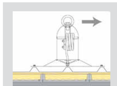
La bobina del Constant Force Post® controla la carga cuando ocurre una caída, limitando el impacto a la cubierta de la construcción.
